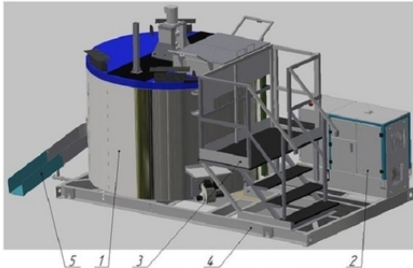
Рисунок – Общий вид оборудования Вулкан 5000
